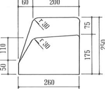
■安全型特殊変形A-1
