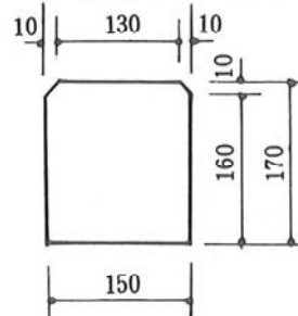
■歩道舗装止縁石
