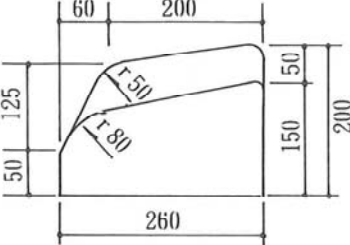
■安全型変形A-2
