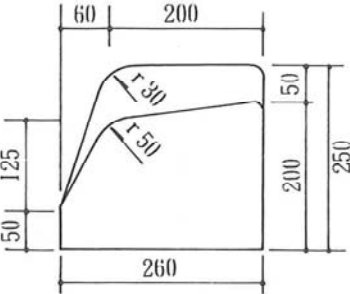
■安全型変形A-1
