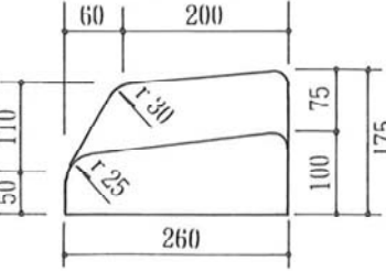
■安全型特殊変形A-2
