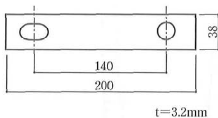
接続金具詳細図
