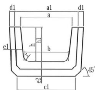
●ソケット部詳細
