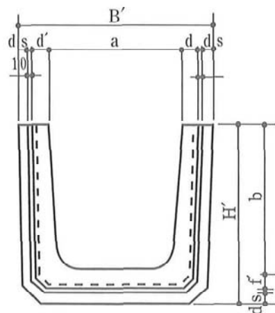
●ソケット部詳細
