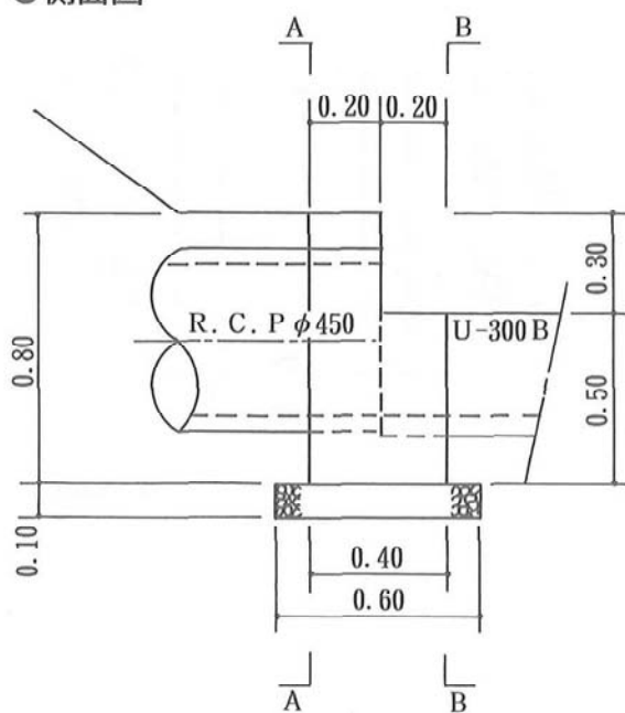
●側面図
