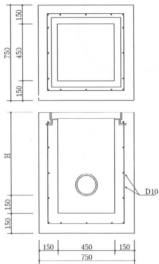
■接続柵(防衛庁タイプ)450
