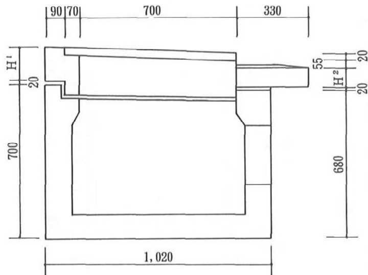
●側面図
