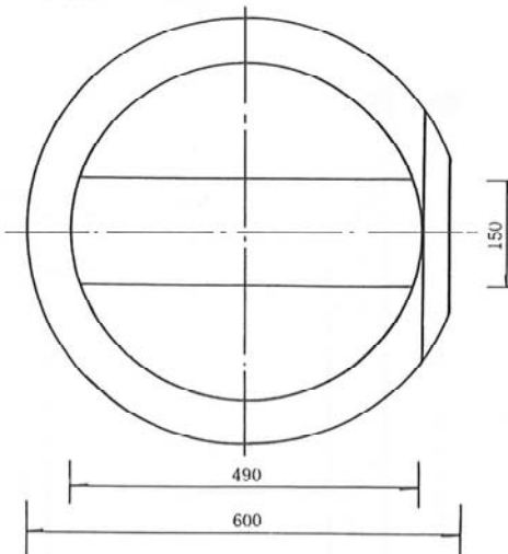
●底部平面図
