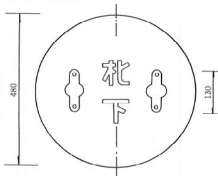
●蓋平面図
