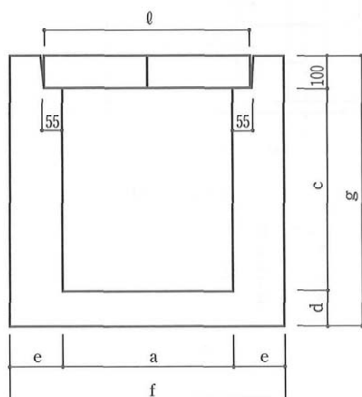
■寸法表
