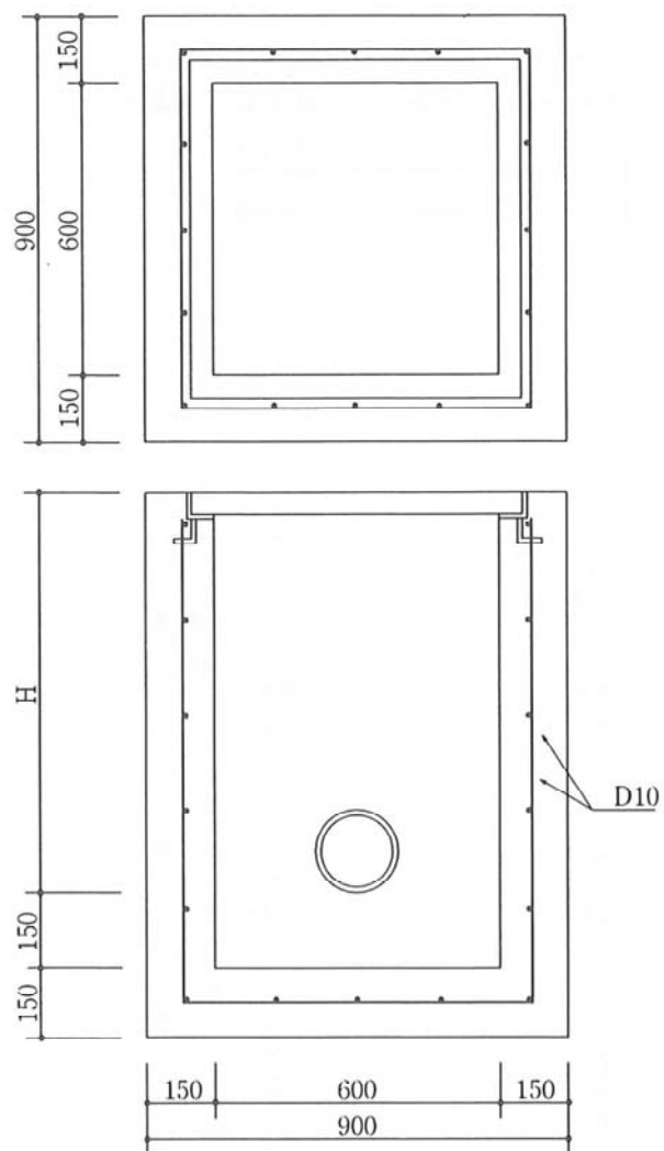
■接続柵(防衛庁タイプ)600
