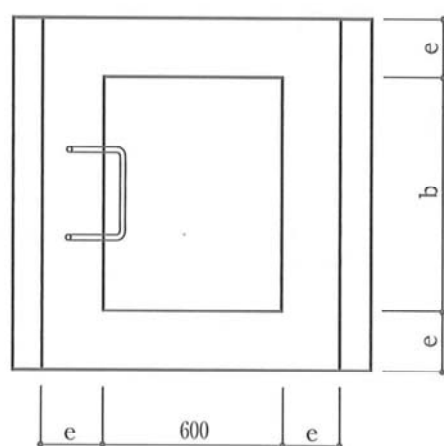
■寸法表
