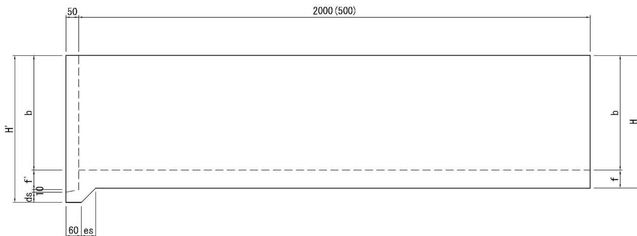
●ソケット部詳細
