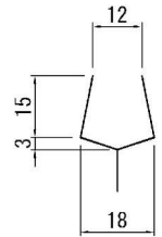
目地の詳細図
