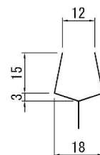
目地の詳細図
