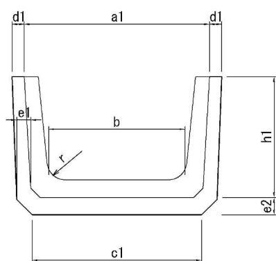
●ソケット部詳細
