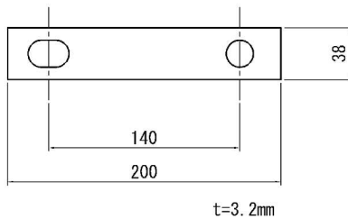
接続金物詳細図
