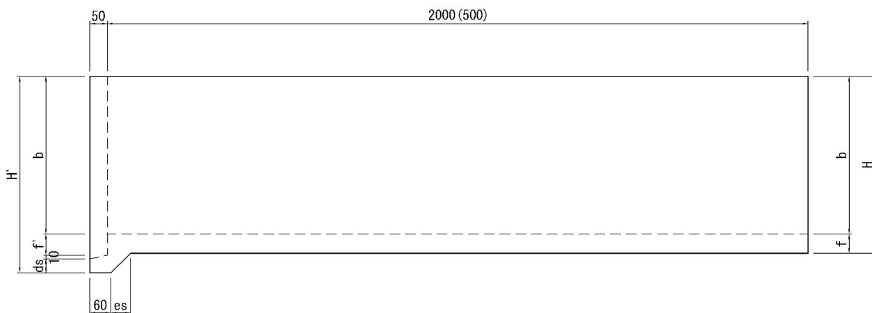
●ソケット部詳細
