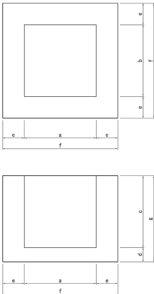
■ 寸法表
