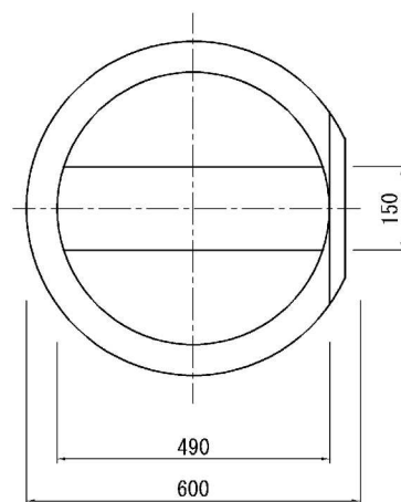
■底部平面図
