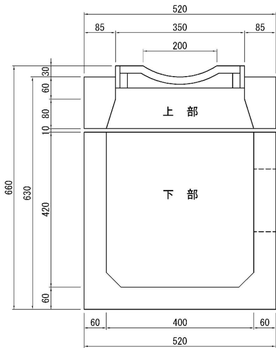
●断面図
