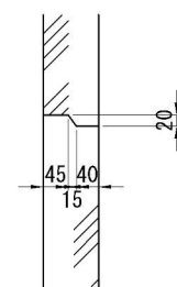
接合部詳細図
