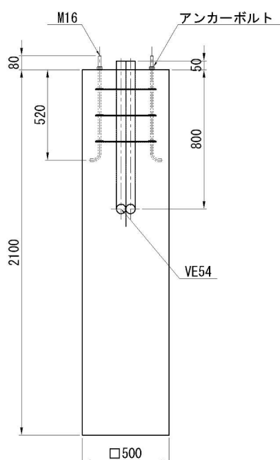
側面図
