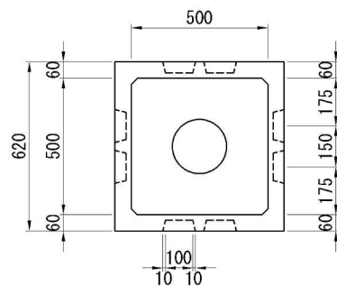
E A型ハンドホール
