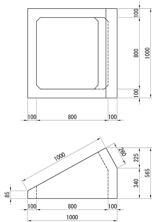
dユニット
