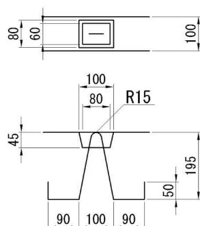
吊り下げフック部詳細
