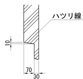
箱抜き部詳細
