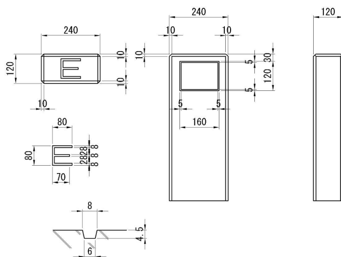
接地埋設標
